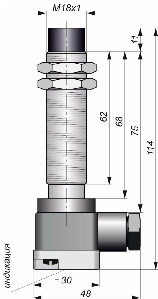
Габаритный чертеж
